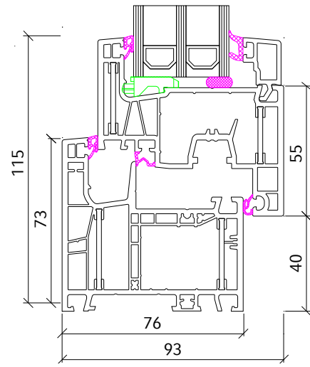
Rahmen 73 mm - Flügel 75 mm
