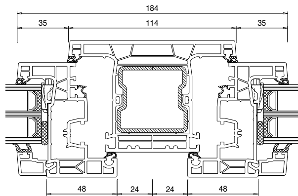
Pfosten 94 mm - Flügel 75 mm
