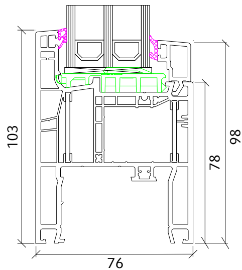
Rahmen 103 mm
